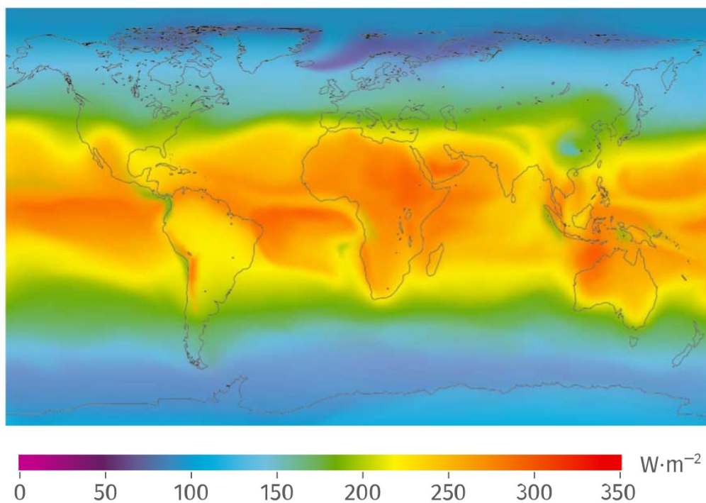
Document n°3 : carte mondiale de l'insolation terrestre (puissance solaire moyenne reçue chaque année par unité de surface)
