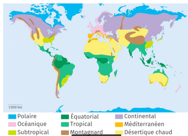
Document n°2 : les ceintures climatiques terrestres
