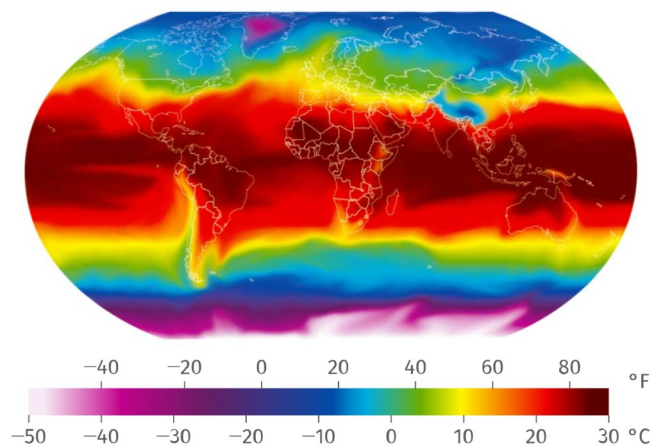
Document n°1 : Planisphère des températures moyennes terrestres
